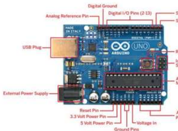
Gambar 4. Arduino Uno (Sumber : http://www.arduino.cc )
