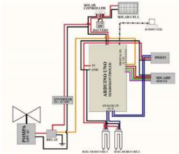
Gambar 1. Skema rangkaian hardware
