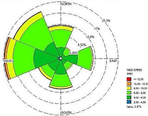
Gambar 4. Windrose Tahun 2011-2020 Tarakan (Sumber : Hasil Analisa Data Menggunakan Software WRPLOT)
