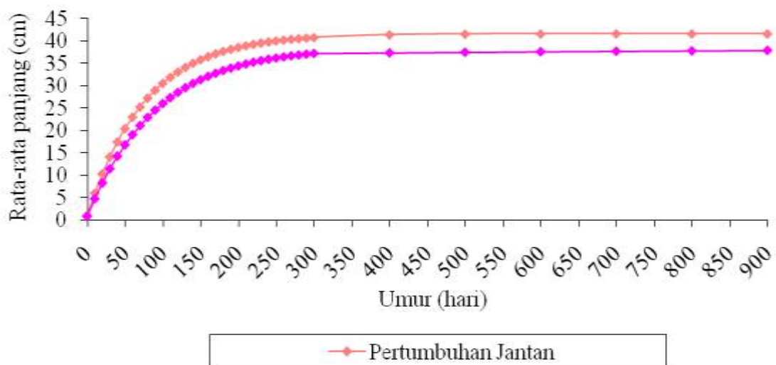
Gambar 1. Kurva Laju Pertumbuhan Ikan puput ( Ilisha elongata )
